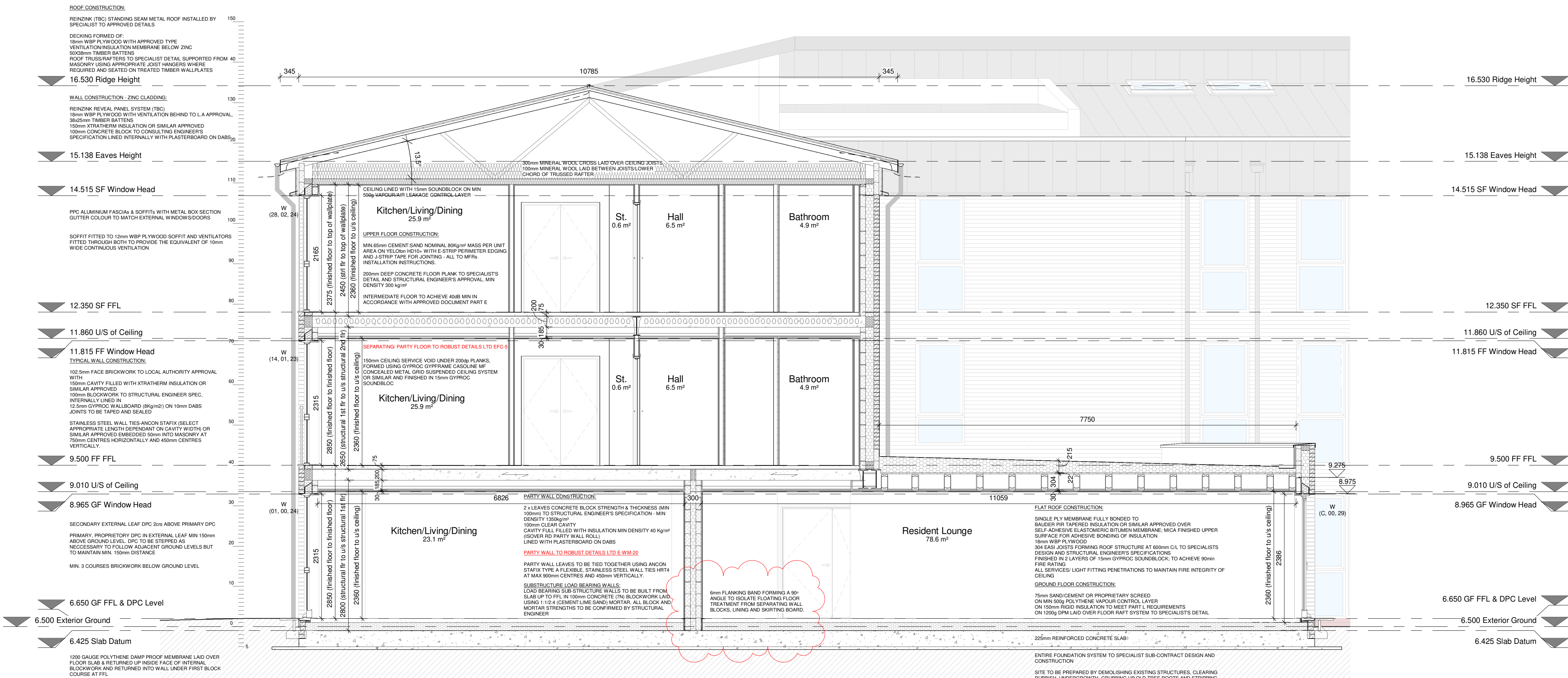
Section BB 1 : 50
