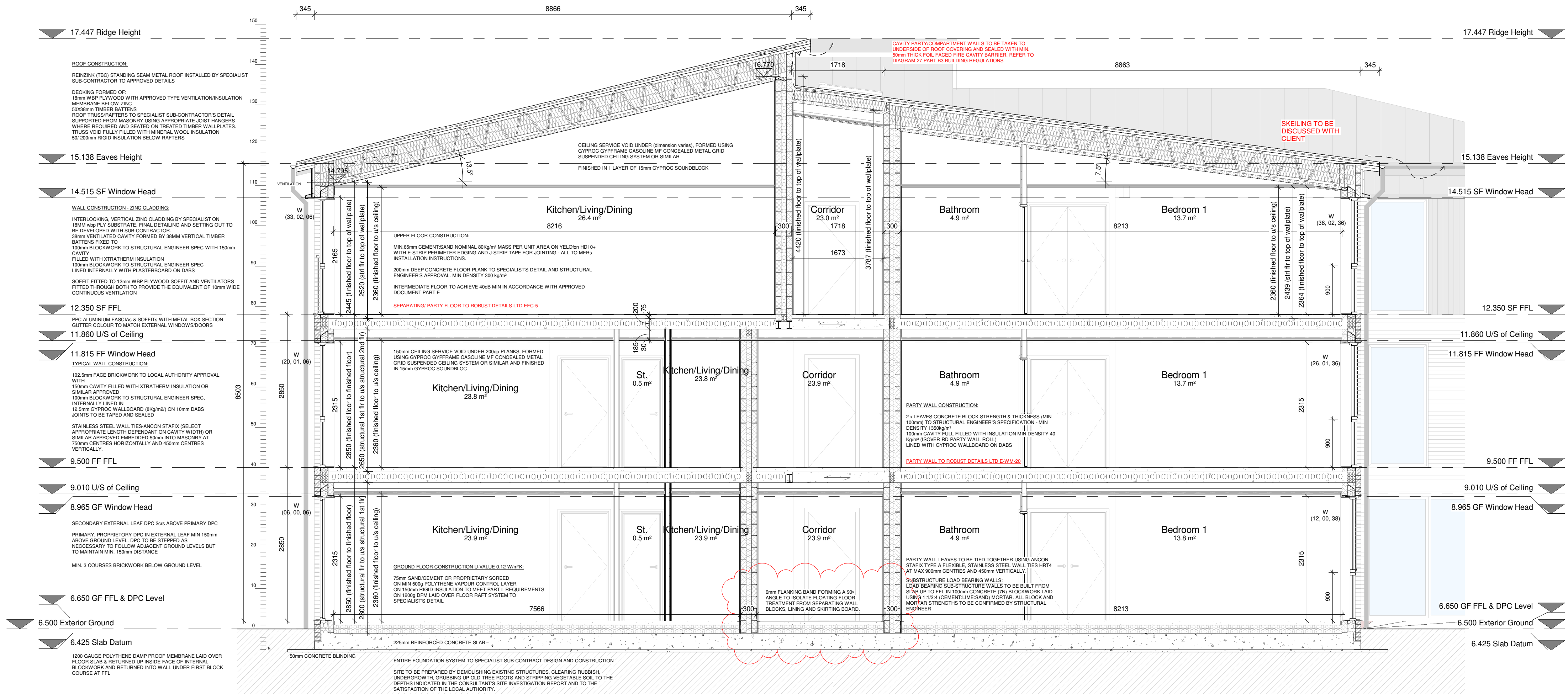
Section AA 1 : 50
