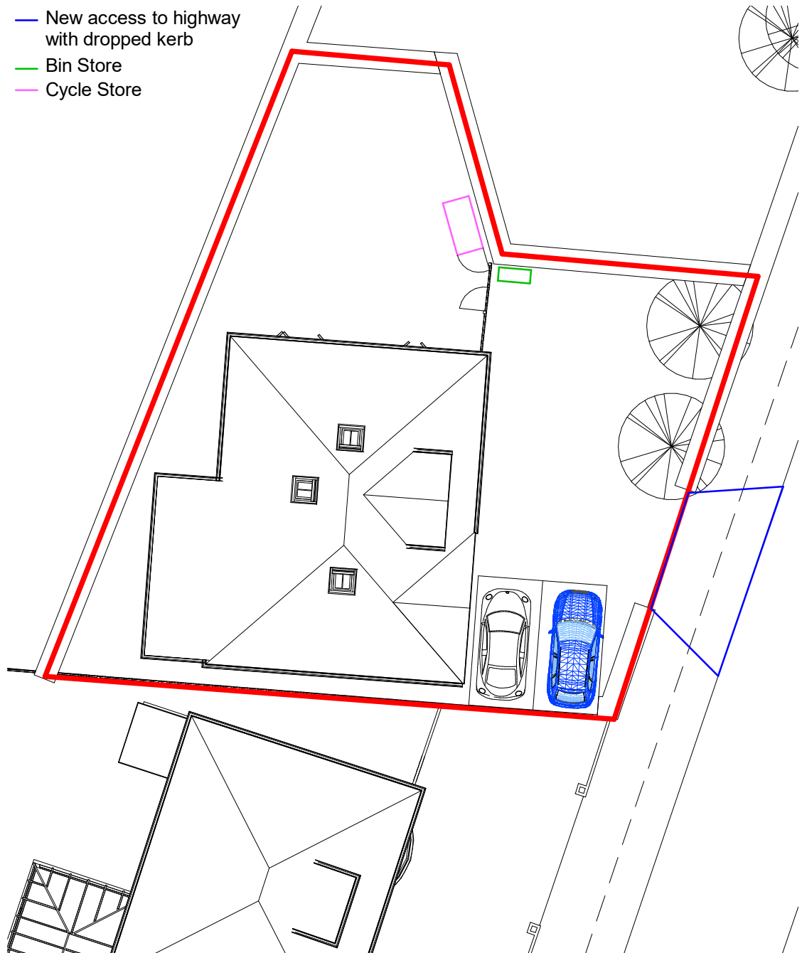
2 Main Site & Roof Plan 1 : 200
