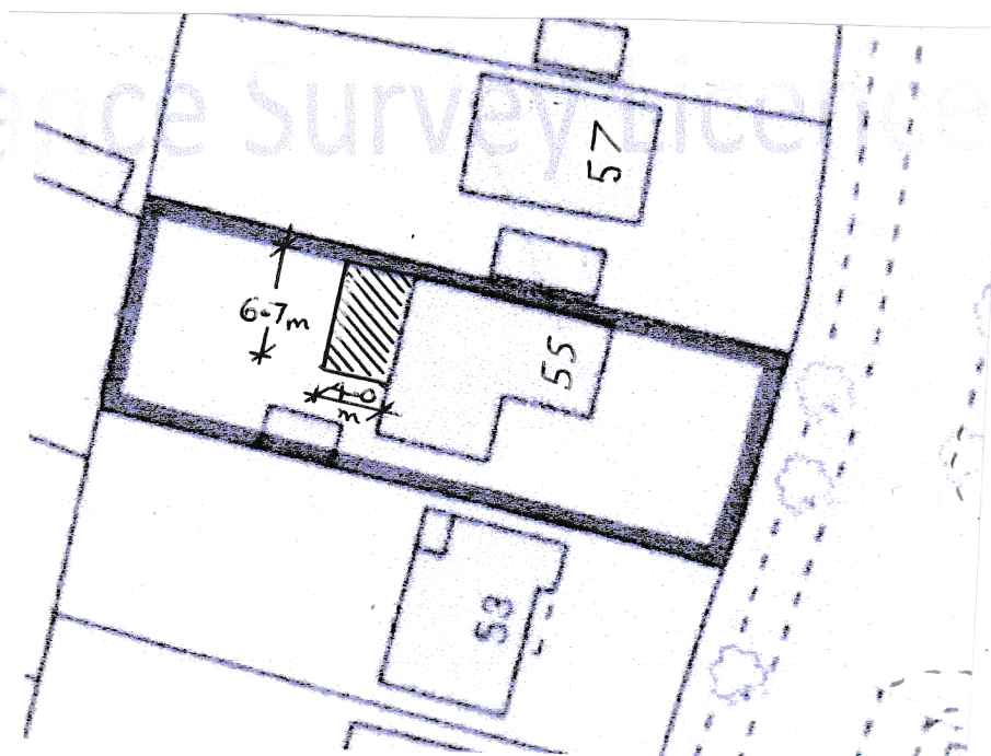
SITE PLAN 1:500
