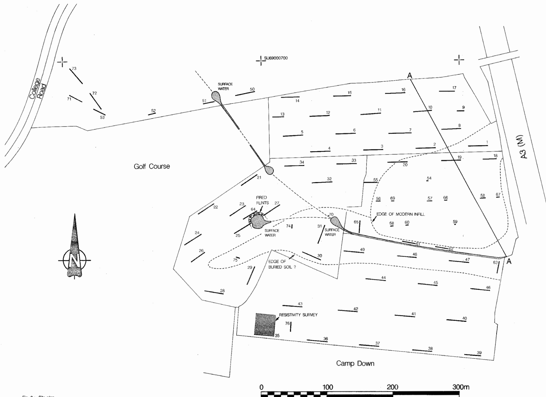
Fig. 2 : Site plan.
