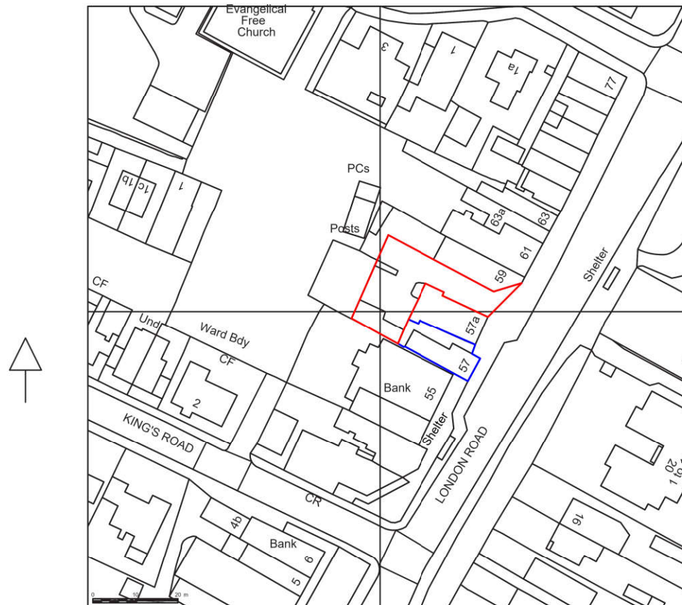
Site Plan @1:1250
