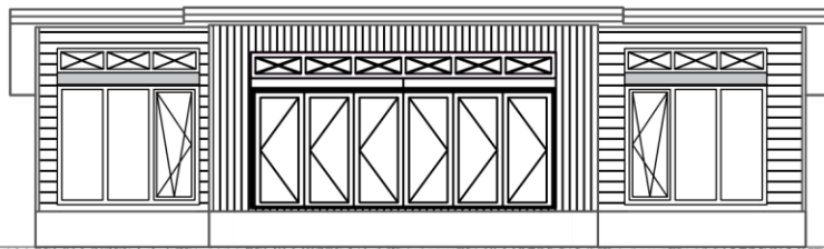
Elevation A
