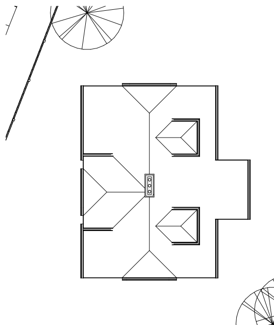
5 Roof Plan 1 : 200
