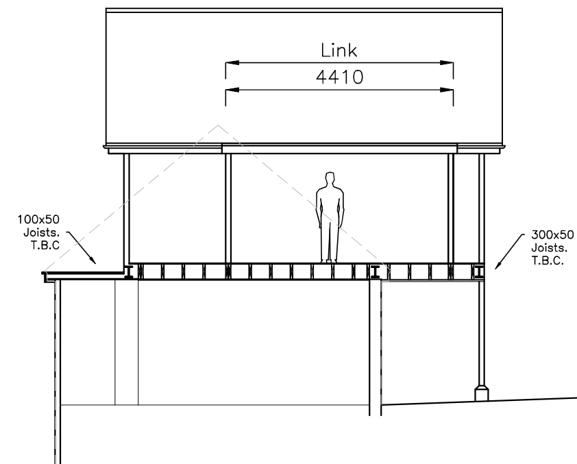
Longitudinal Section
