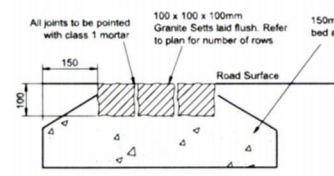
GRANITE SETTS RUMBLE STRIP 3 ROWS (Scale 1:10)
