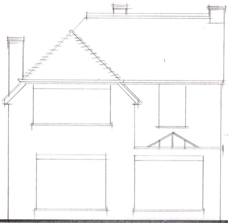
SE elevation
