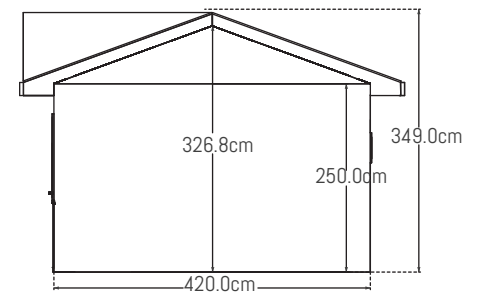
Right elevation
