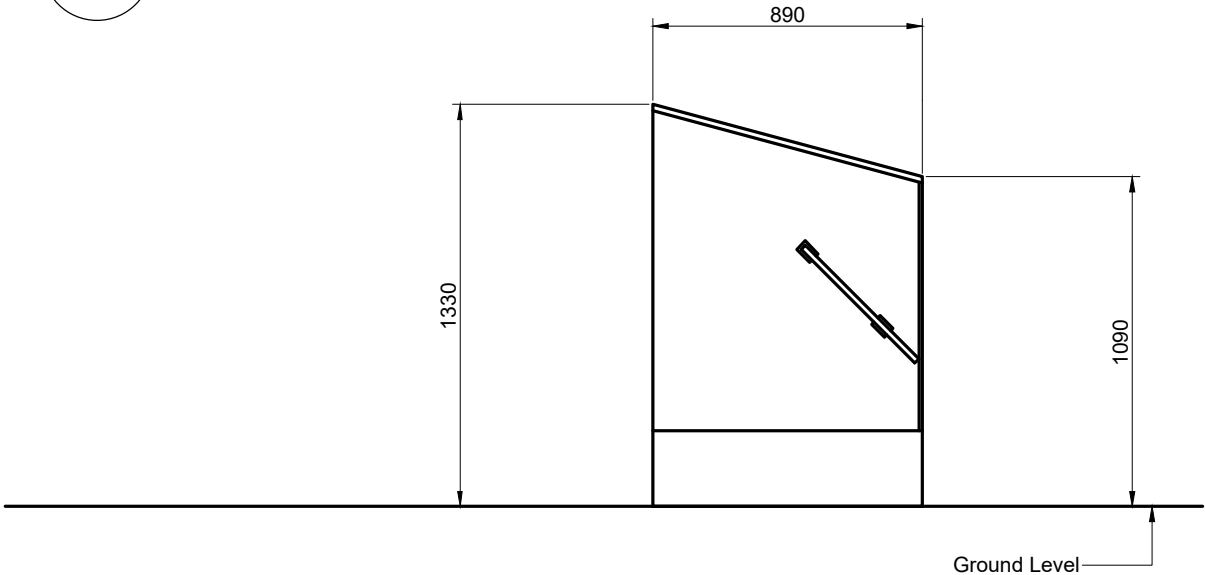
01 Elevation - Side D02 1:25 @ A3
