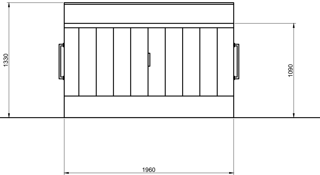
04 Elevation - Front D02 1:25 @ A3
