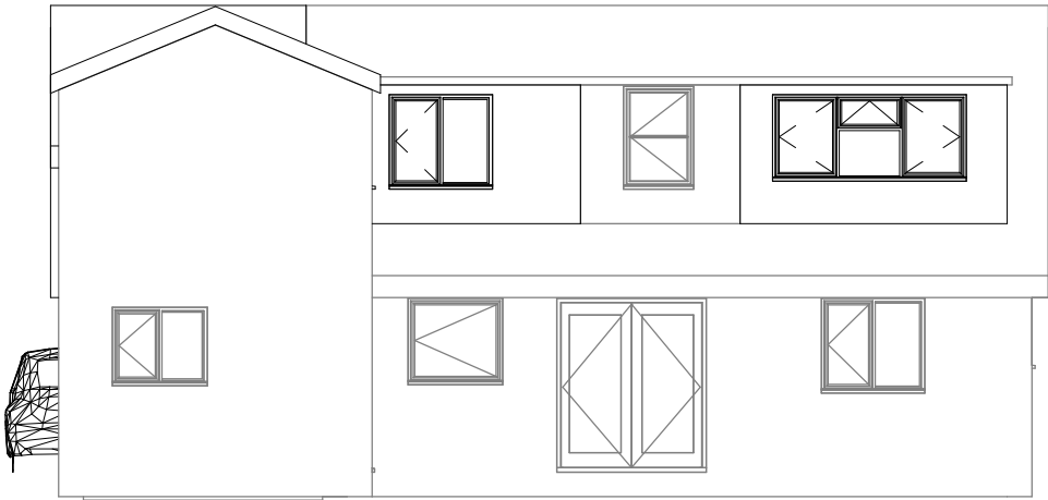
2 East 1 : 100
