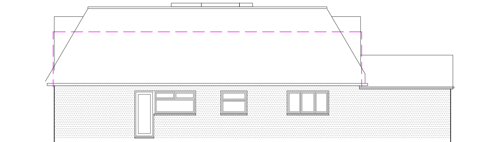
SIDE (E) 1:100
