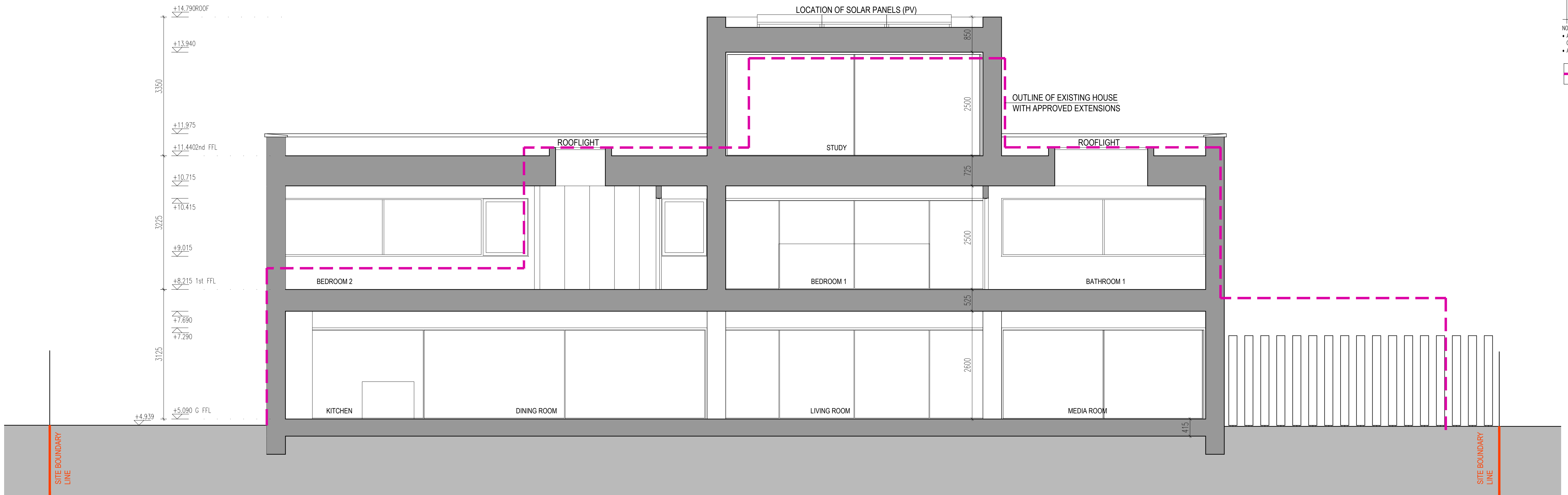
SECTION A-A
