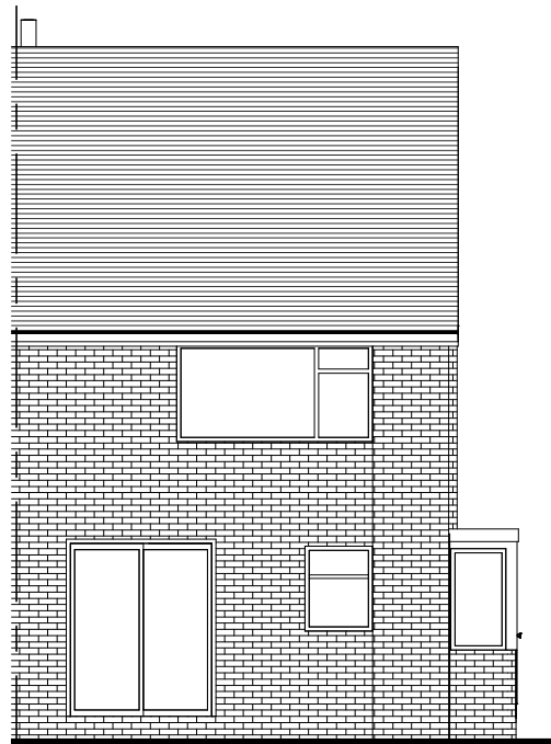
Existing SE Elevation
