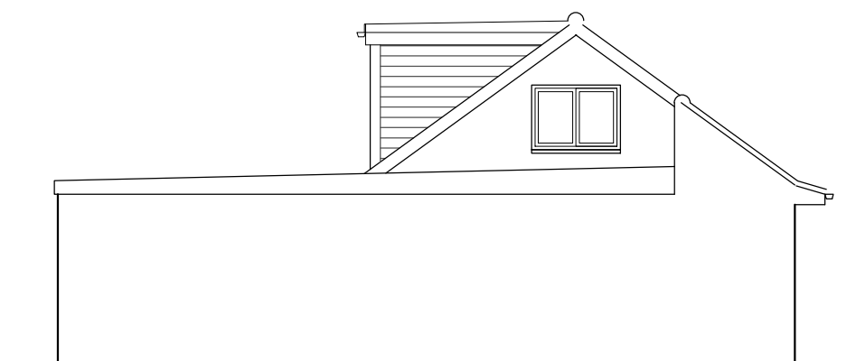
SIDE (N) 1:100
