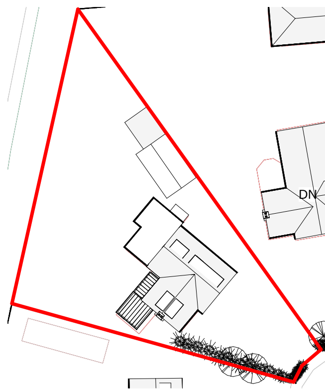
2 Site Plan 1 : 500
