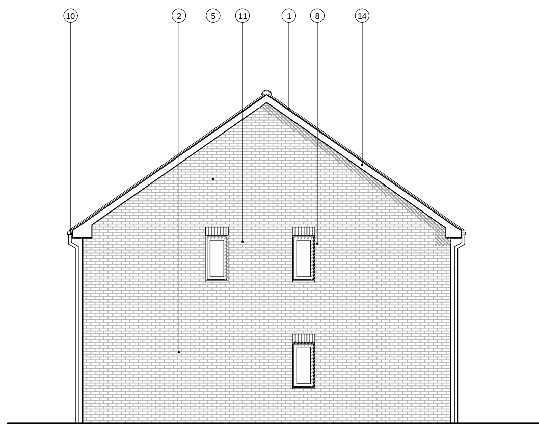
07 Elevation 04 2005 Scale: 1:100
