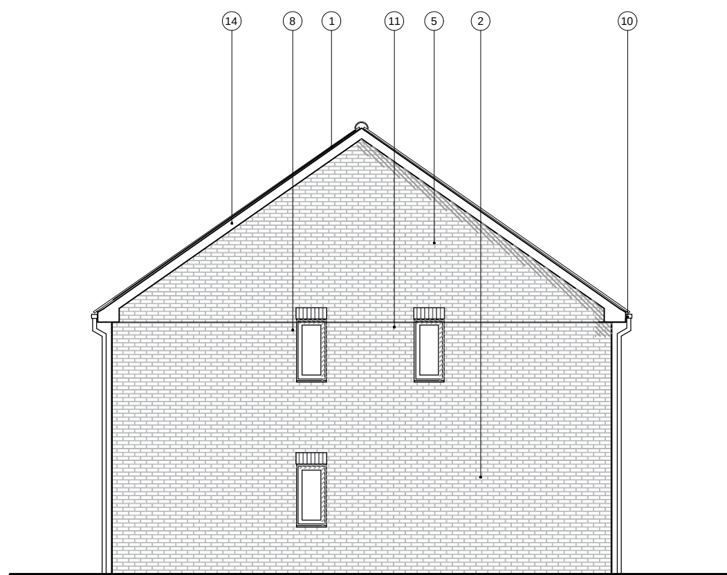
06 Elevation 03 2005 Scale: 1:100
