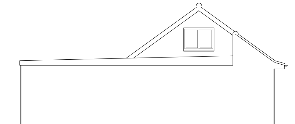
SIDE (N) 1:100
