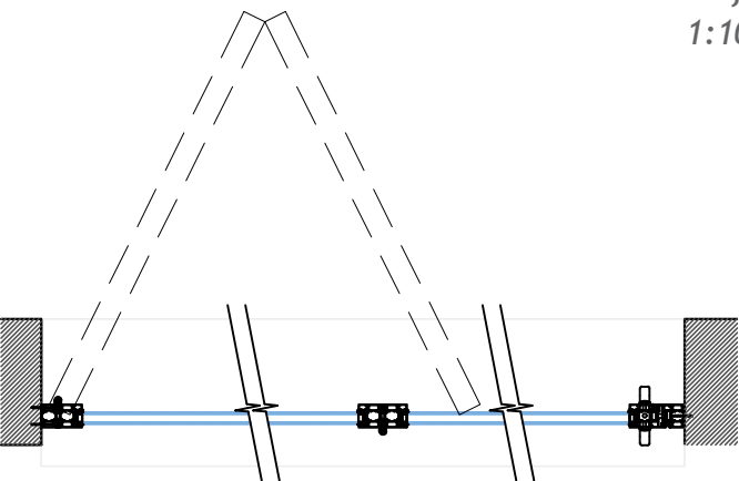
Door Plan Aluminium Frame Bi-fold 1:20
