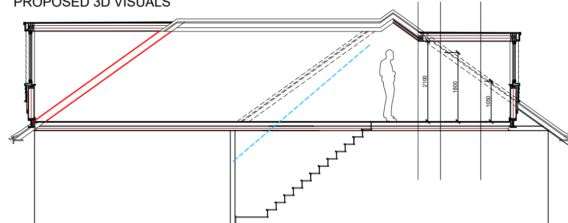
SECTION B-B scale 1:200 @ A3 1:100 @ A1
