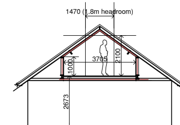
SECTION A-A scale 1:200 @ A3 1:100 @ A1
