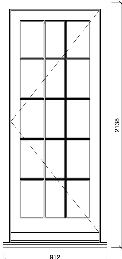
Door D.02 1:20
