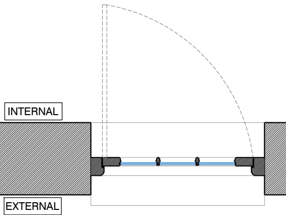
Door Plan 1:20
