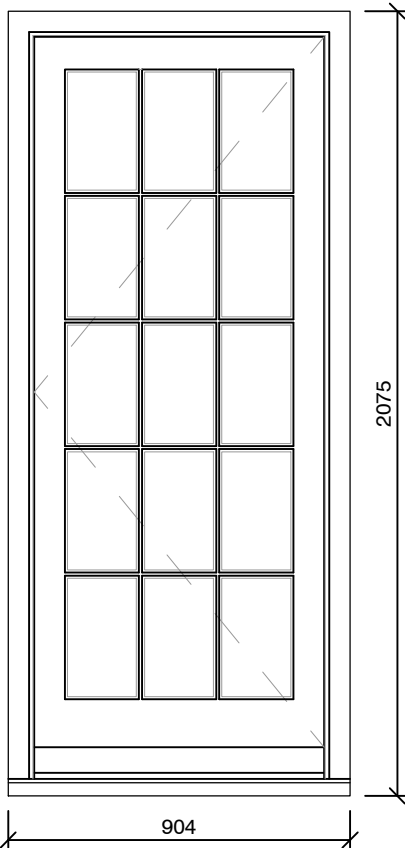
Door D.01 1:20
