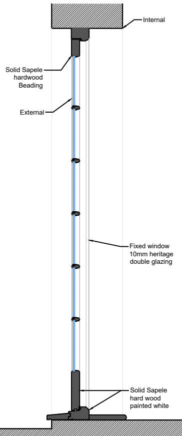
Door Section 1:20
