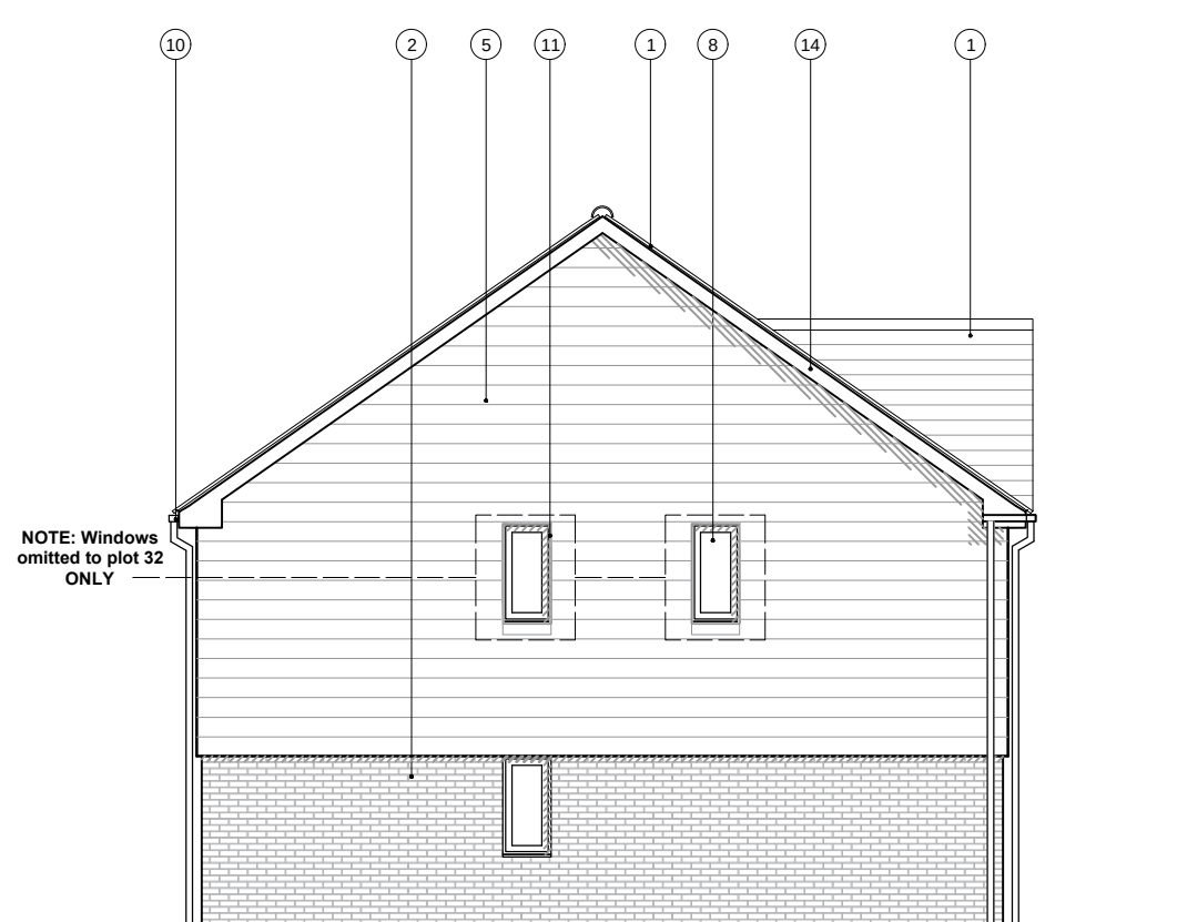
07 Elevation 04 2004 Scale: 1:100
