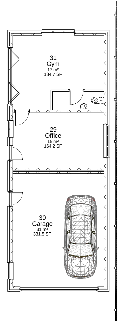
1 Garage Floor Plan 1 : 100
