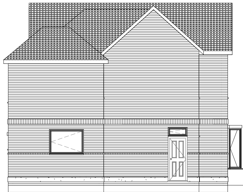
1 West 1 : 100
