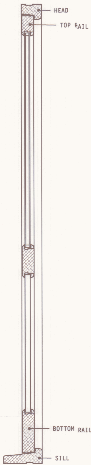
typical door vert section
