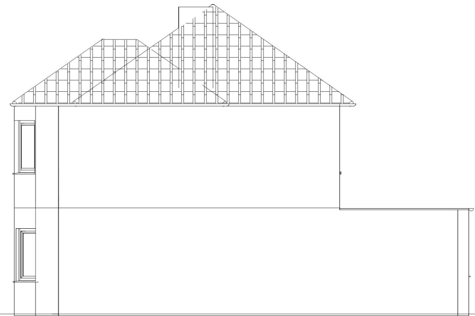
Right Elevation
