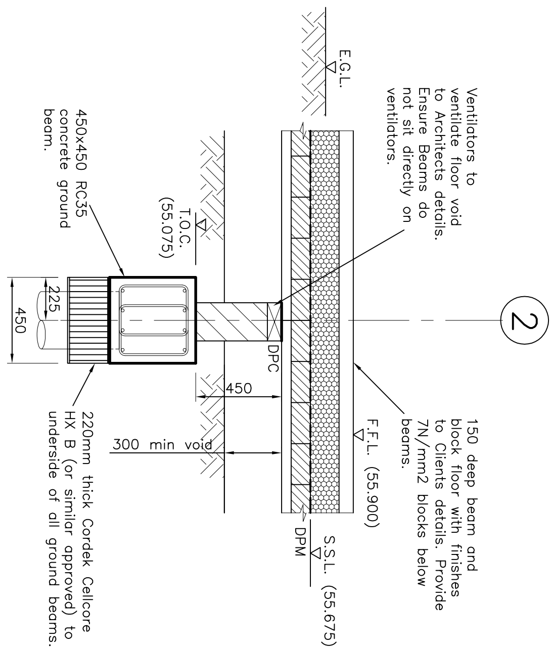
SECTION E-E 1:20
