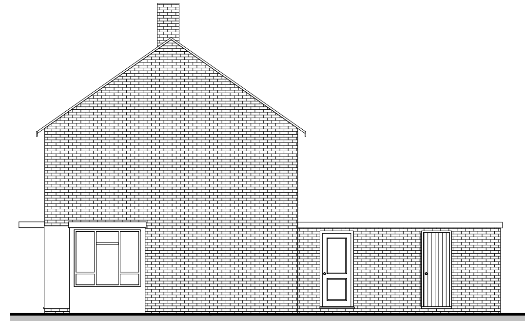
Existing SE Elevation
