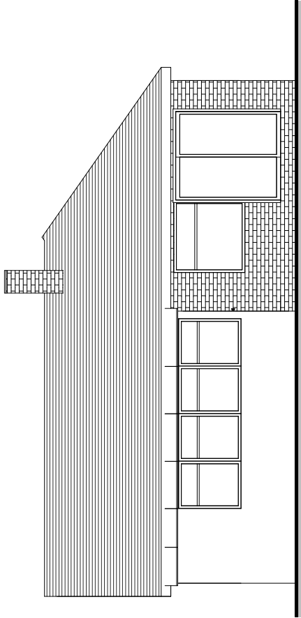
Existing SE Elevation 1 : 100
