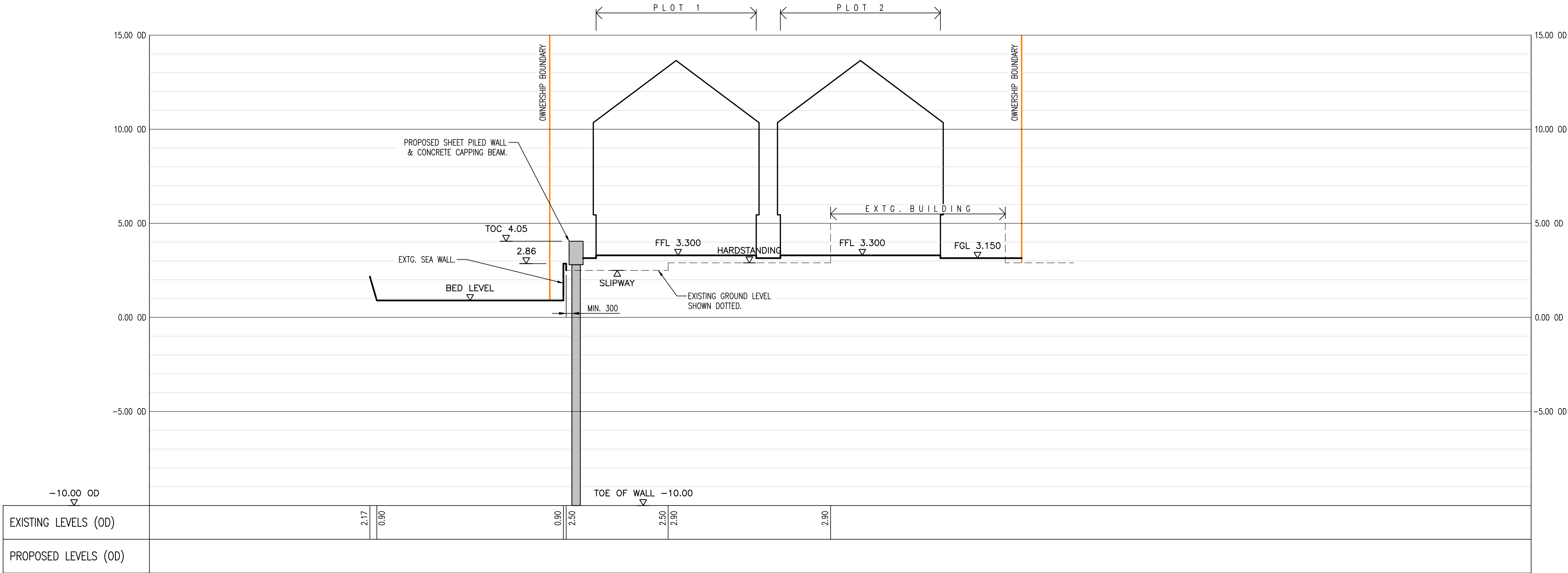
SECTION A-A. SCALE 1:125
