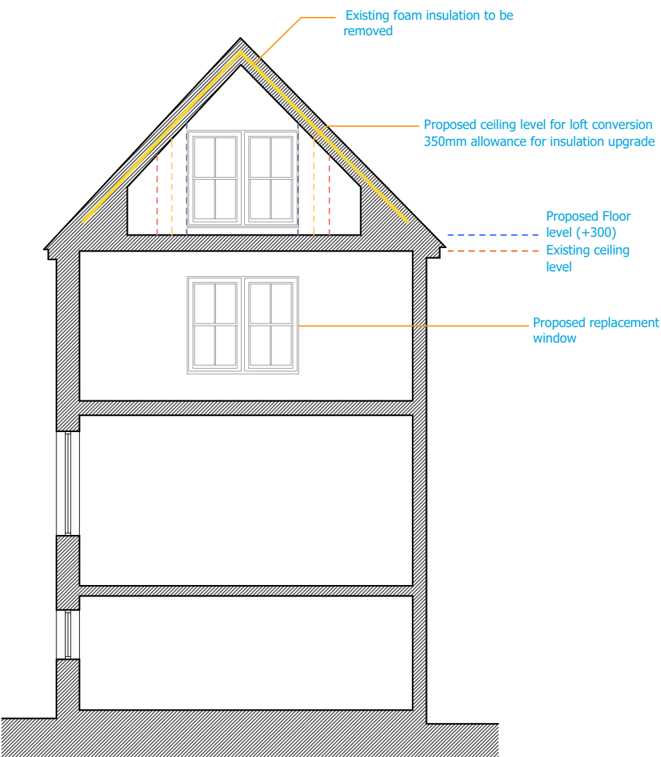
SECTION A-A 1:100
