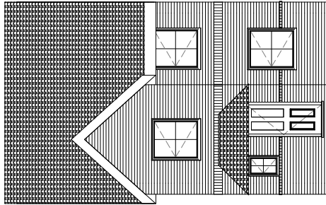
2 South 1 : 100
