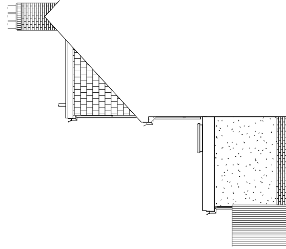
ELEVATION SIDE - NE 1 : 100
