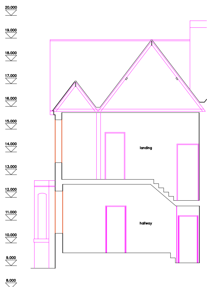
Section A-A 1:100
