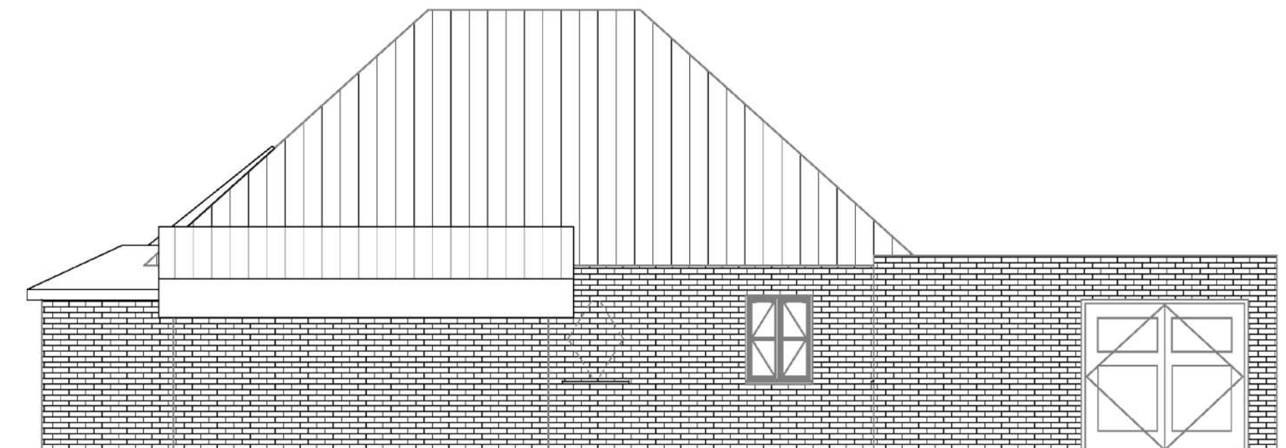
3 North 1 : 100
