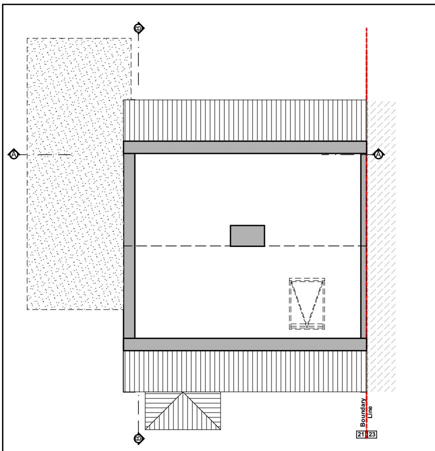
Loft Plan
