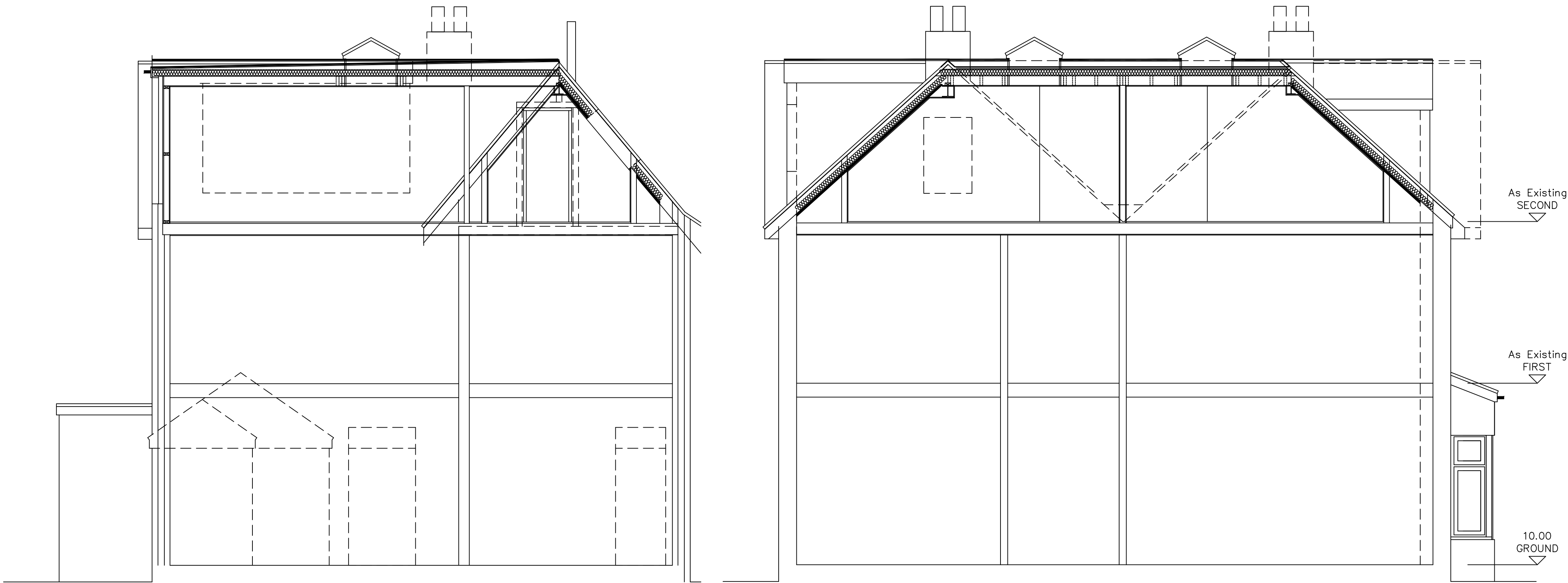
SECTION A-A SCALE 1 : 50
