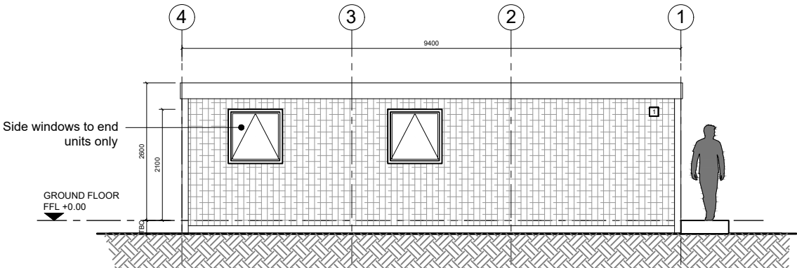
elevation 3-3
