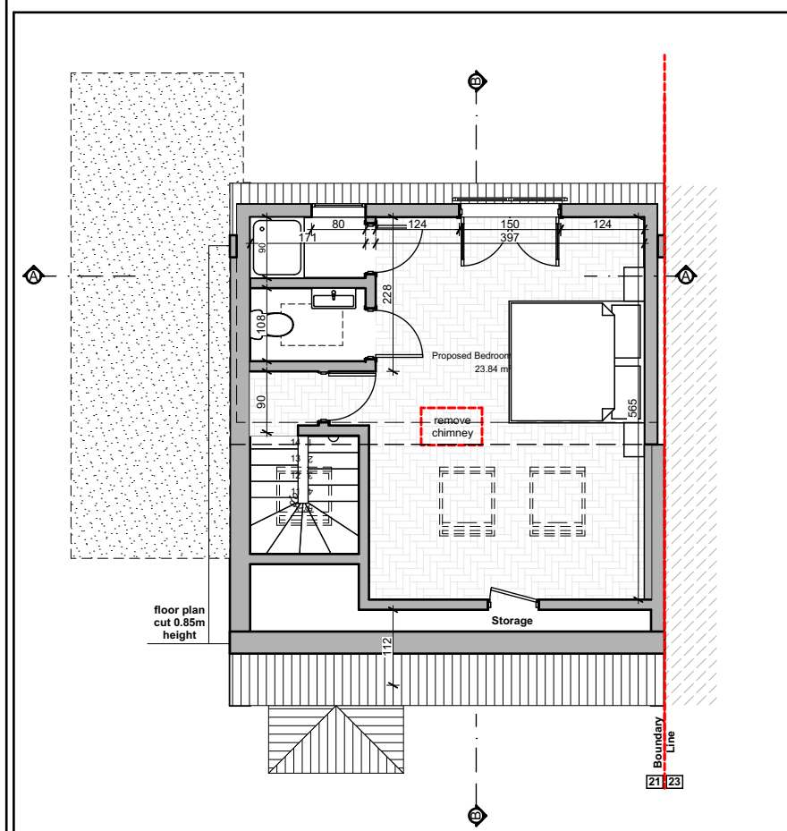
Loft Plan
