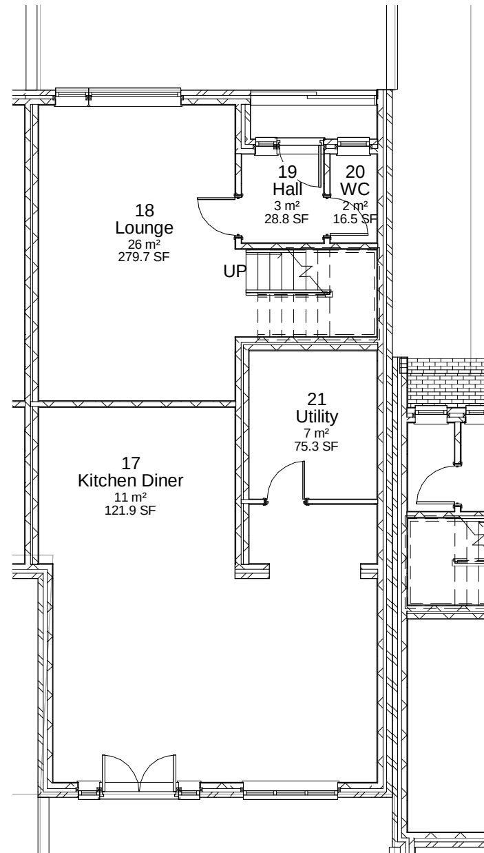
1 Ground - 40A 1 : 100
