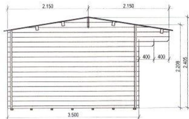
Elevation 6
