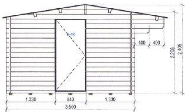
Elevation 5
