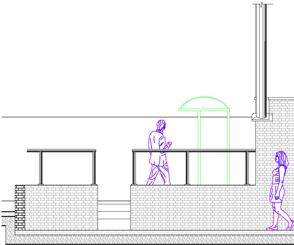
Elevation B - B' Scale 1:50
