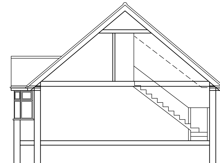
SECTION A-B
