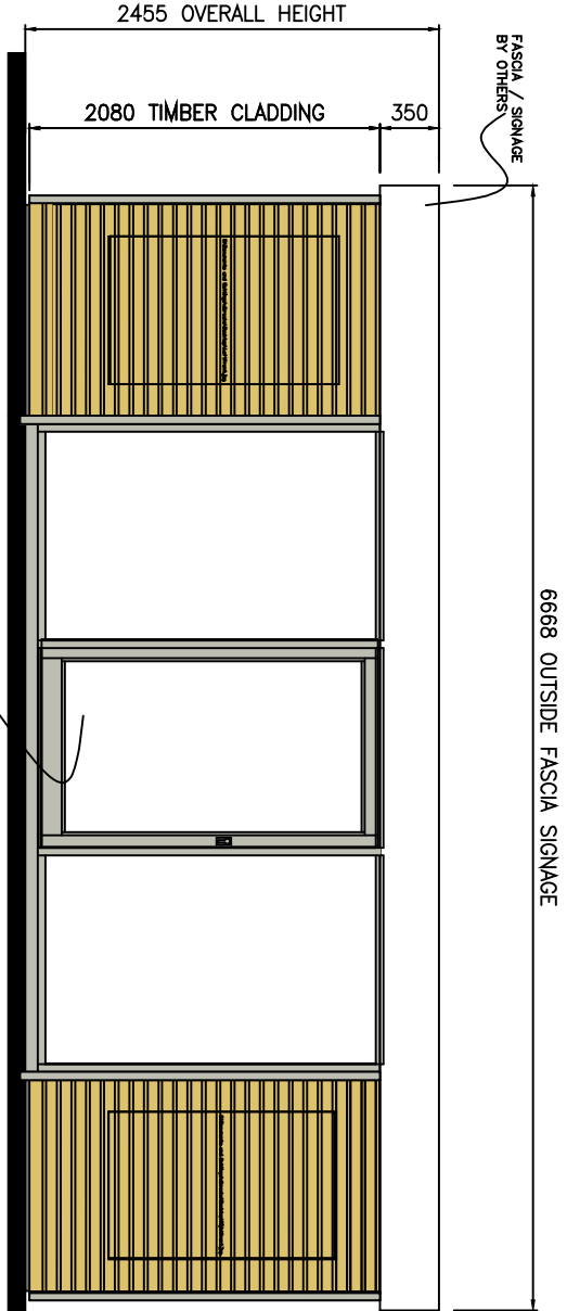
ELEVATION A-A
