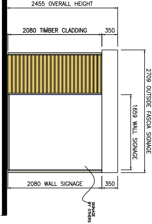
ELEVATION B-B
