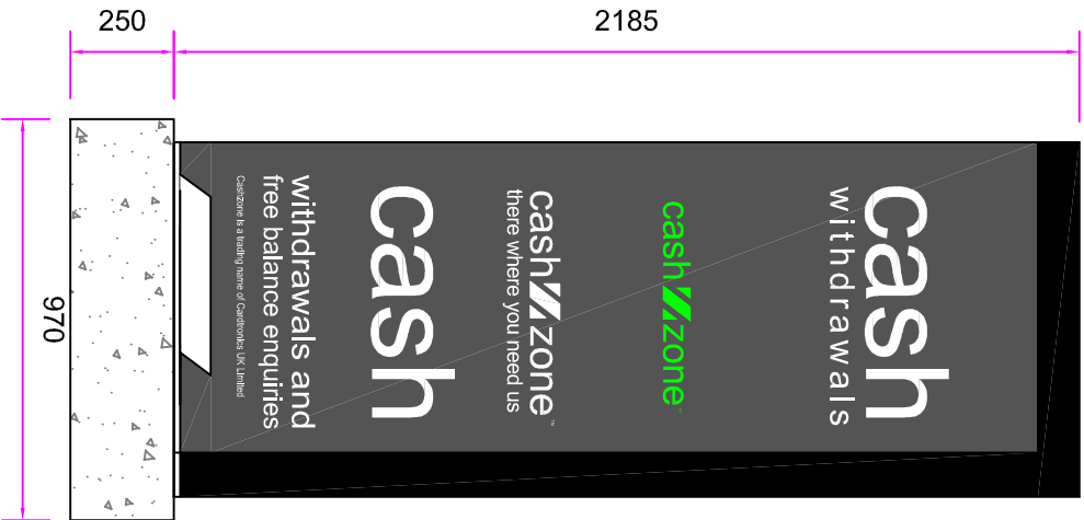
L/H/S ELEVATION - BODEX POD w/NCR 6622e ATM
