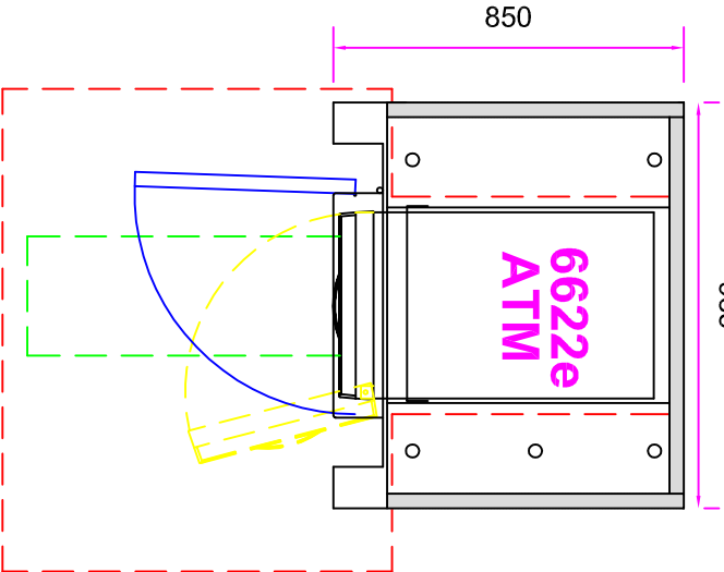
PLAN - BODEX POD w/NCR 6622e ATM
