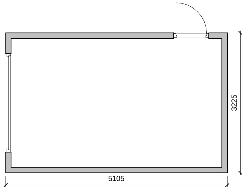
5 Garage Floor Plan 1 : 50
