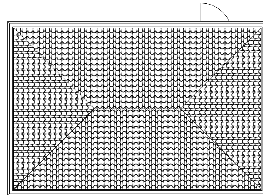
6 Garage Roof Plan 1 : 50
