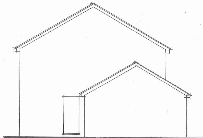
SIDE ELEVATION - N.
