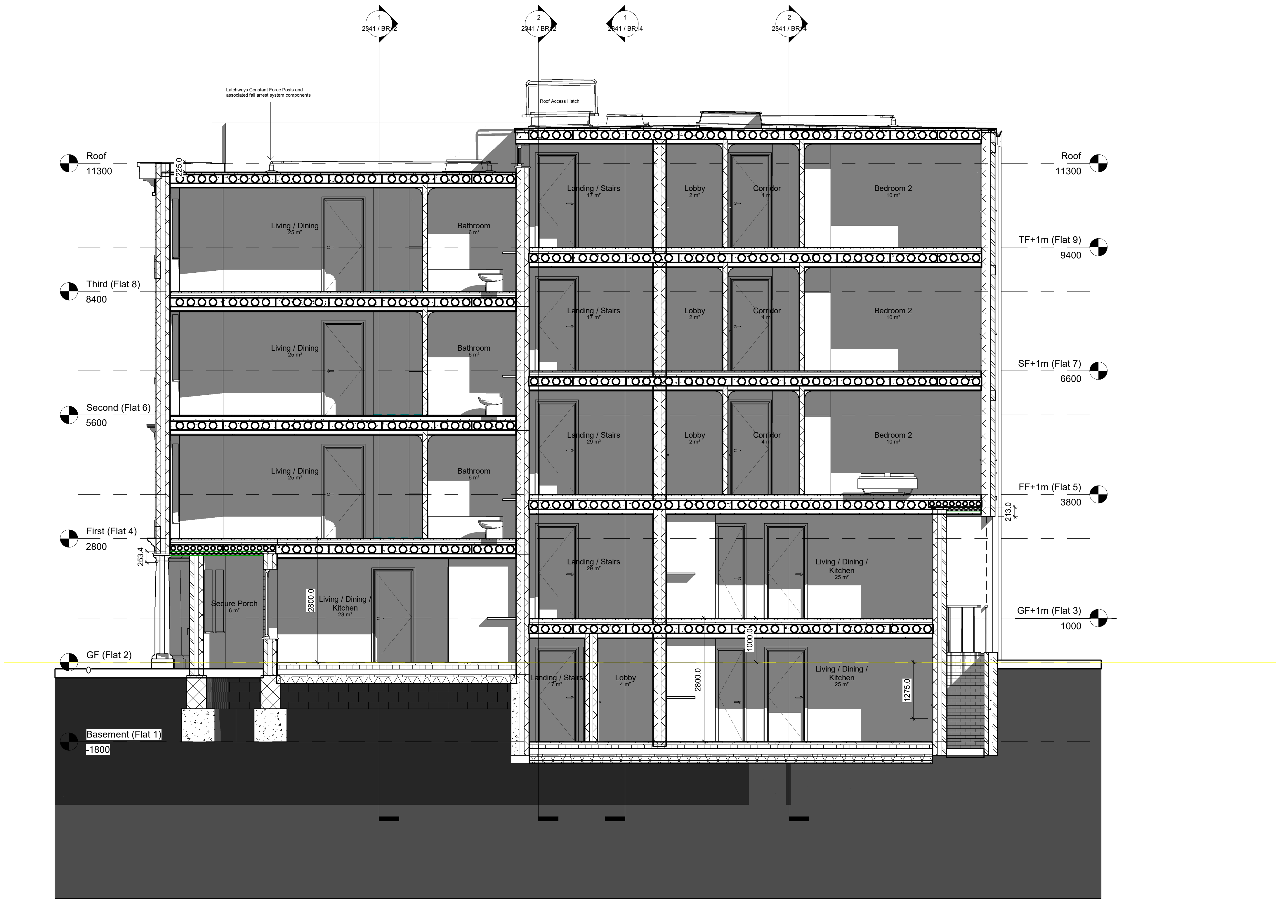
Section AA 1 : 50
